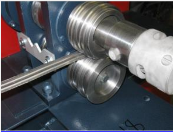
изготовление хомутов
